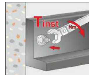
Serrer au couple indiqué dans les données de montage
